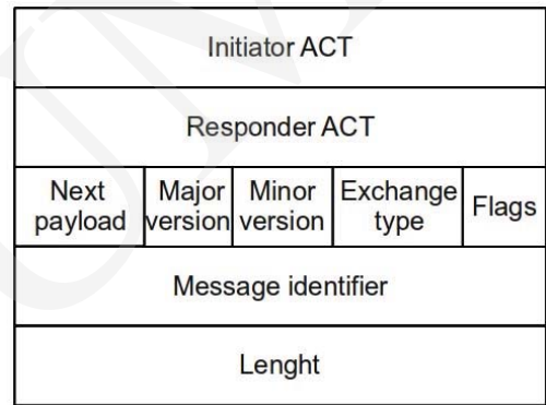
Fig. 2. ISAKMP header.
