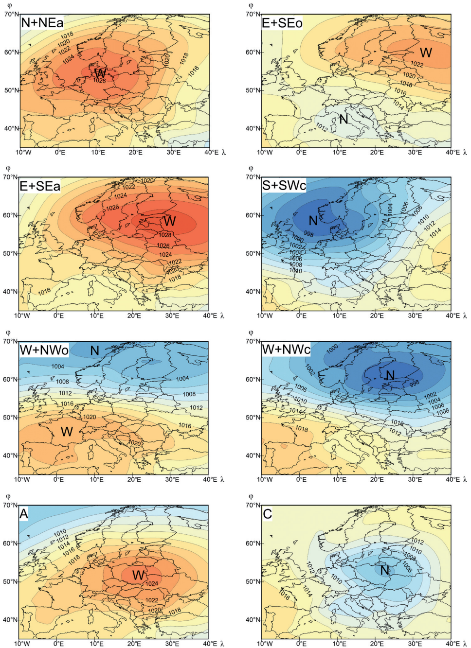
Ryc. 1. Średnie pole ciśnienia atmosferycznego na poziomie morza (hPa) nad Europą podczas występowania wybranych typów cyrkulacji w okresie 1951–2010
