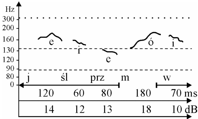
Rys. 15. Tonogram wypowiedzenia jeśli przemówi . Niski żeński głos KB
